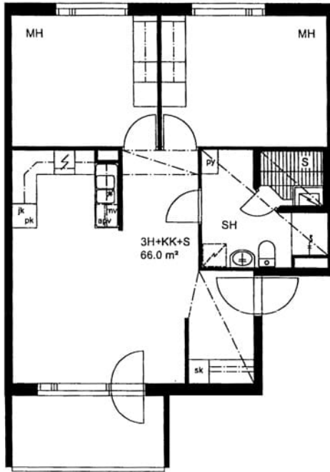
Vasamakuu 5-7 B 26 / pohjakuva Not in scale
