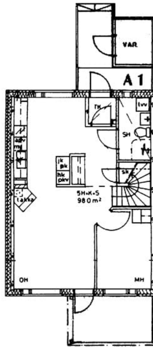
Viertopolku 1 A1 / pohjakuva 1. kerros Ei mittakaavassa
