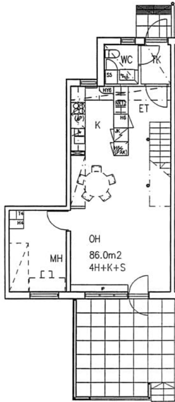
Lippukatu 5 B 10 / pohjakuva 1. kerros Ei mittakaavassa
