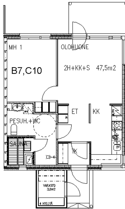
Pajaharjuntie 2 C 10 / pohjakuva
