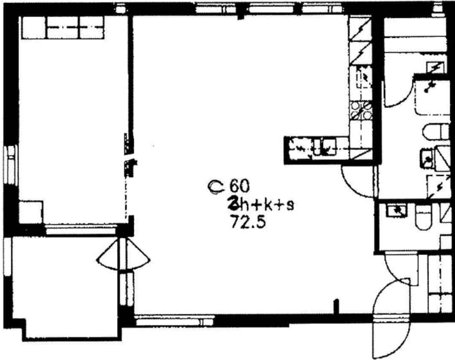
Mustankivenaukio 3 C 60 / pohjakuva
