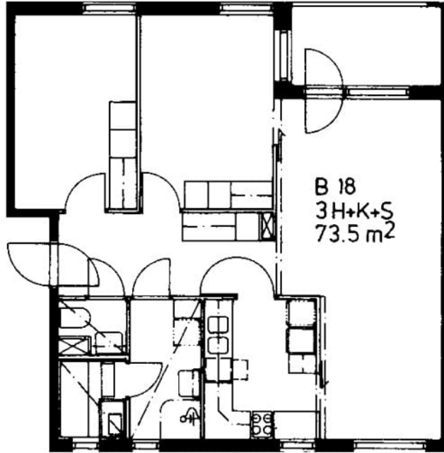
Ruutikuja 1 B 18 / pohjakuva Not in scale
