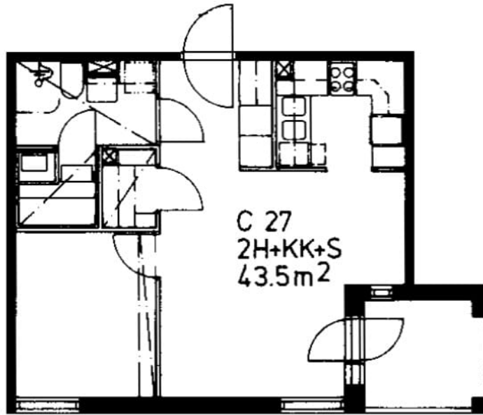
Ruutikuja 1 C 27 / pohjakuva Ei mittakaavassa
