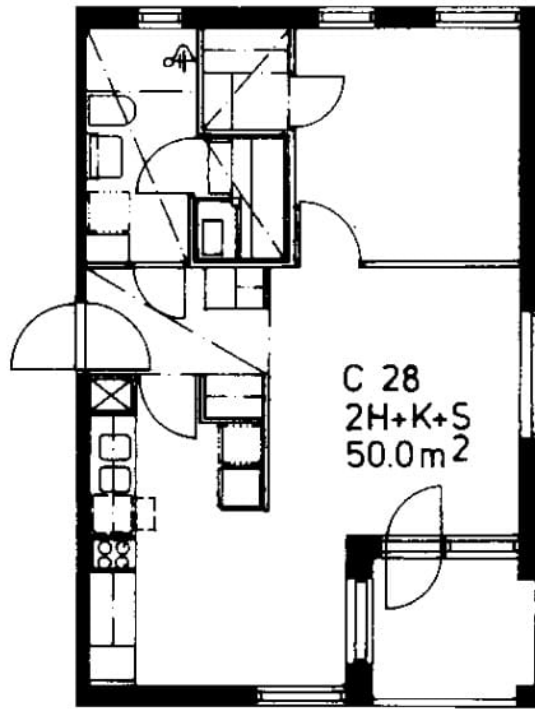
Ruutikuja 1 C 28 / pohjakuva Not in scale
