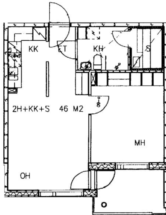
Trillakatu 2 B 18 / pohjakuva Ei mittakaavassa
