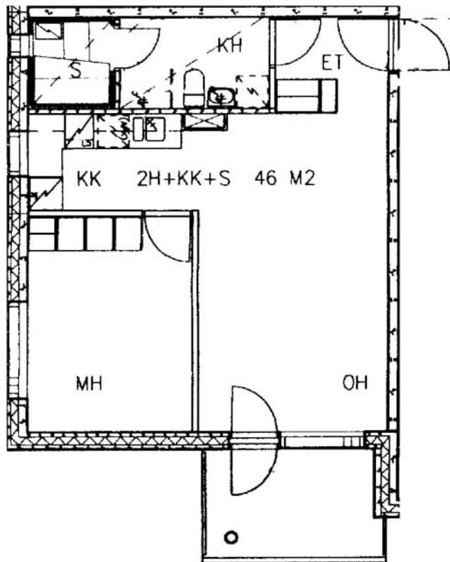
Trillakatu 2 A 6 / pohjakuva Ei mittakaavassa
