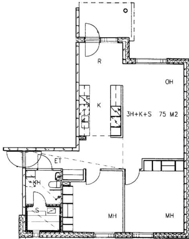
Trillakatu 2 D 47 / pohjakuva Not in scale
