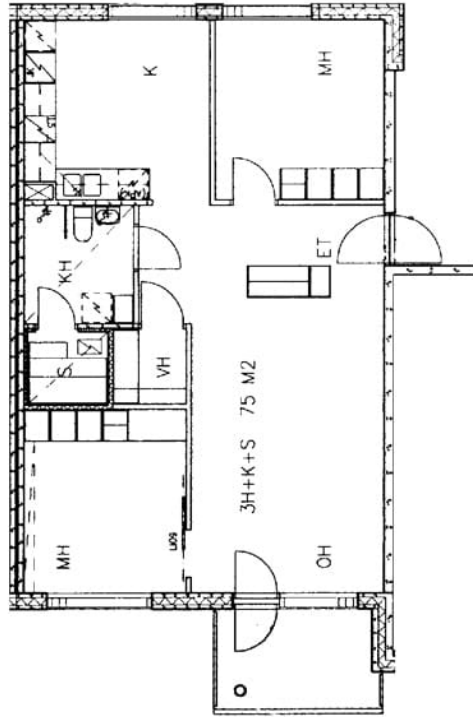
Trillakatu 2 C 31 / pohjakuva Ei mittakaavassa
