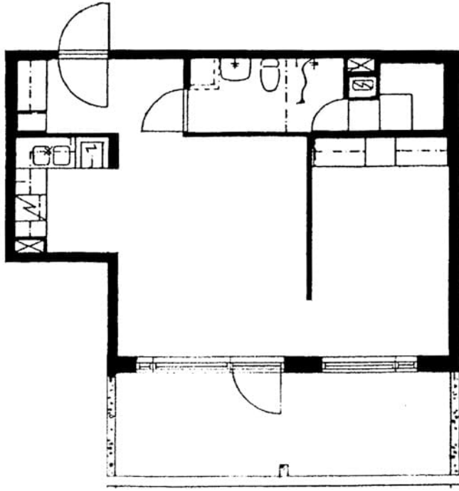
Punamäenpolku 1 B 14 / pohjakuva Ei mittakaavassa
