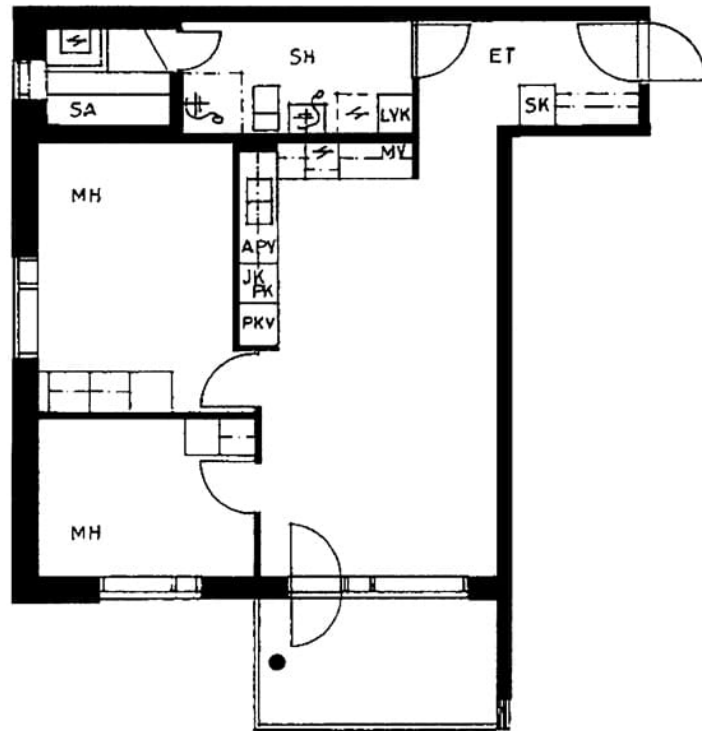
Hernekuja 2 A 3 / pohjakuva Not in scale
