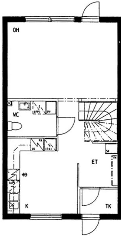
Jokipellonkatu 5 D 12 / pohjakuva 1. kerros Not in scale
