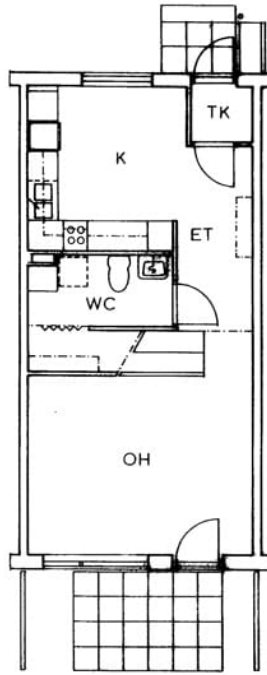
lestie 2 C 8 / pohjakuva 1. kerros
