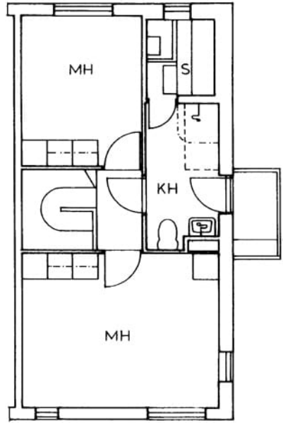
lestie 1 B 3 / pohjakuva 2. kerros
