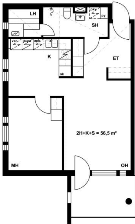
Pikkulukontie 1 B 21 / Pohjakuva
