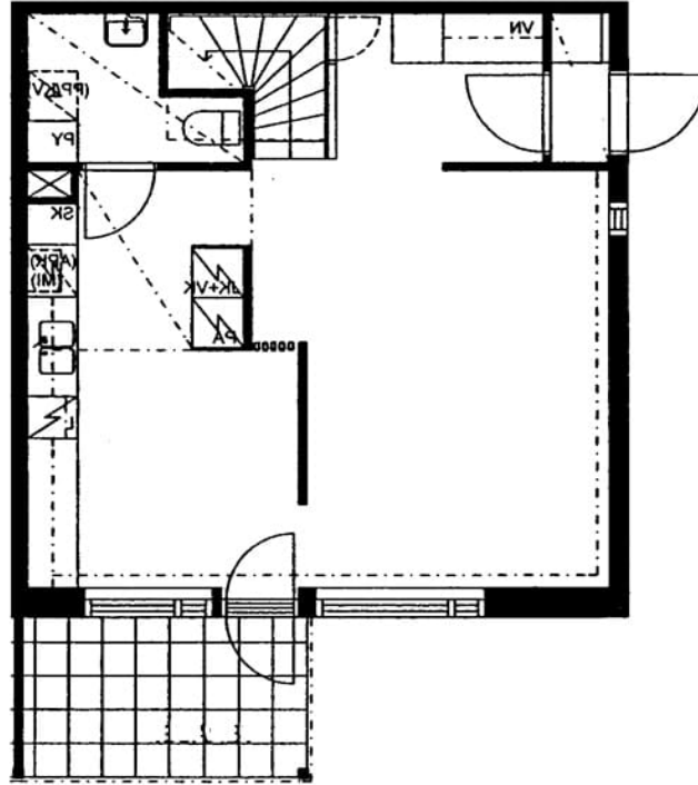
Ruutikuja 8 B 5 / pohjakuva 1.kerros Not in scale
