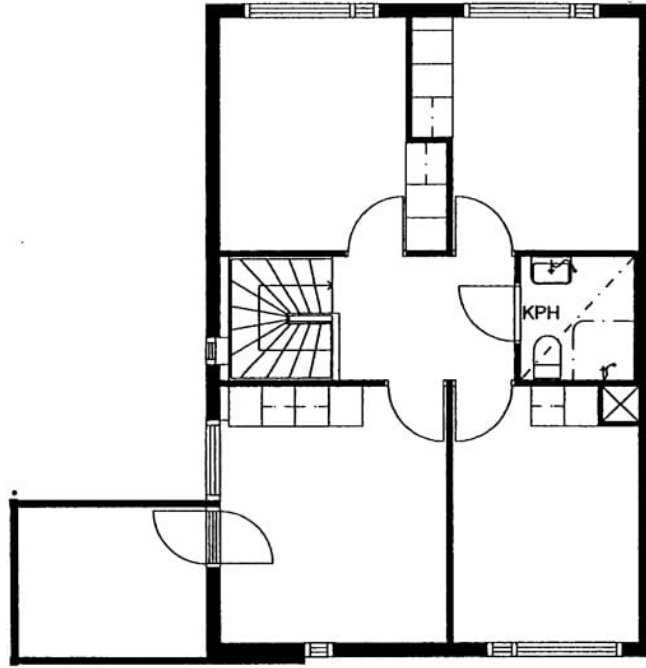
Ruutikuja 5 D 18 / pohjakuva 2.kerros Not in scale
