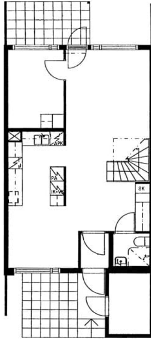
Ruutikuja 5 E 24 / pohjakuva 1.kerros Not in scale
