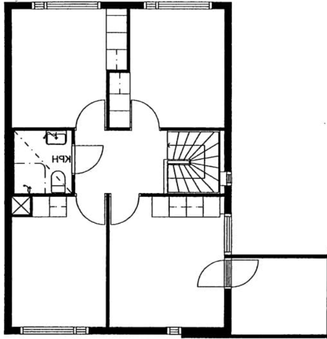
Ruutikuja 5 E 25 / pohjakuva 2.kerros Not in scale
