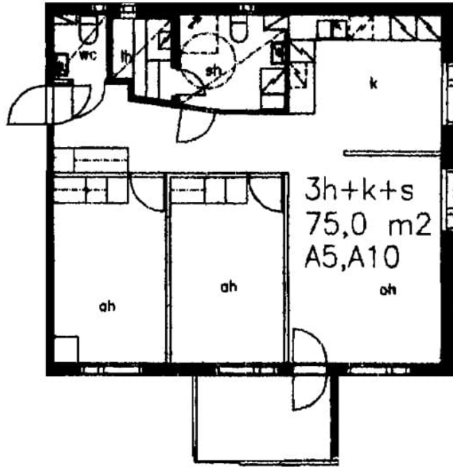
Joupinkuja 2 A 10 / pohjakuva Not in scale
