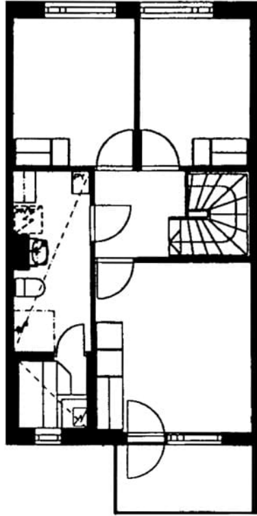
Hallainvuorentie 5 G 27 / pohjakuva 2. kerros Ei mittakaavassa
