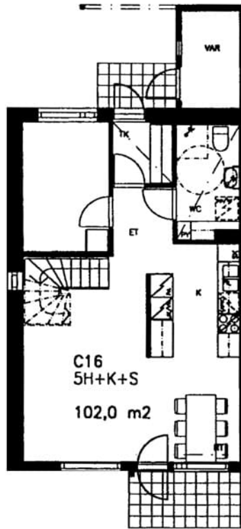
Hallainvuorentie 5 E 20 / pohjakuva 1. kerros Not in scale
