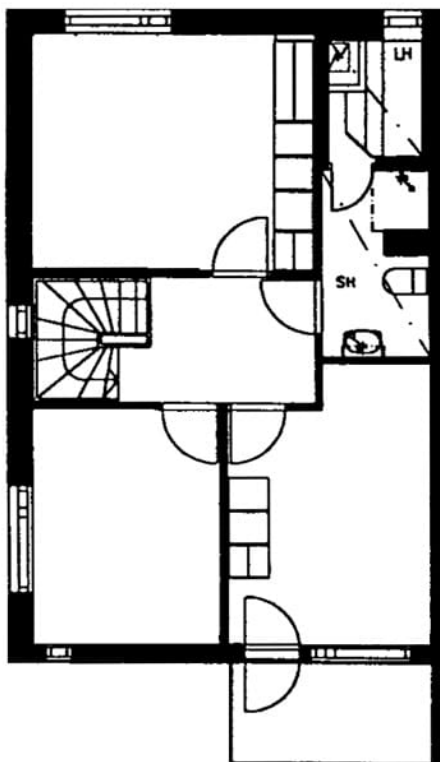
Hallainvuorentie 5 E 20 / pohjakuva 2. kerros
