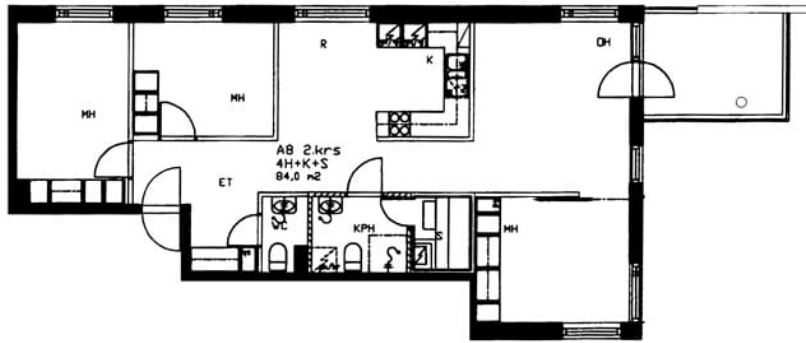
Nappulakatu 2 A 8 / pohjakuva Ei mittakaavassa
