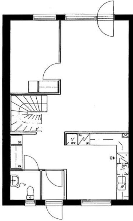
Leppälinnuntie 22 A 1 / pohjakuva 1. kerros Not in scale
