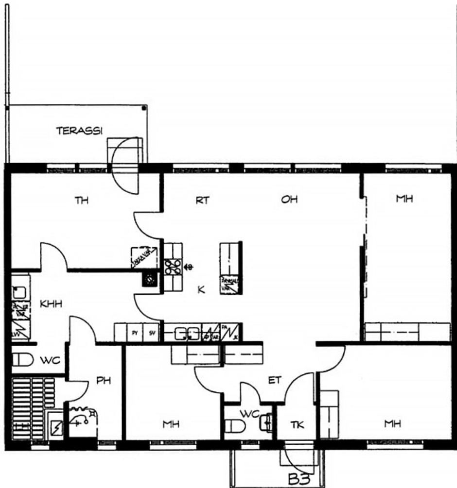
Ullantie 29B B 3 / Pohjakuva Ei mittakaavassa
