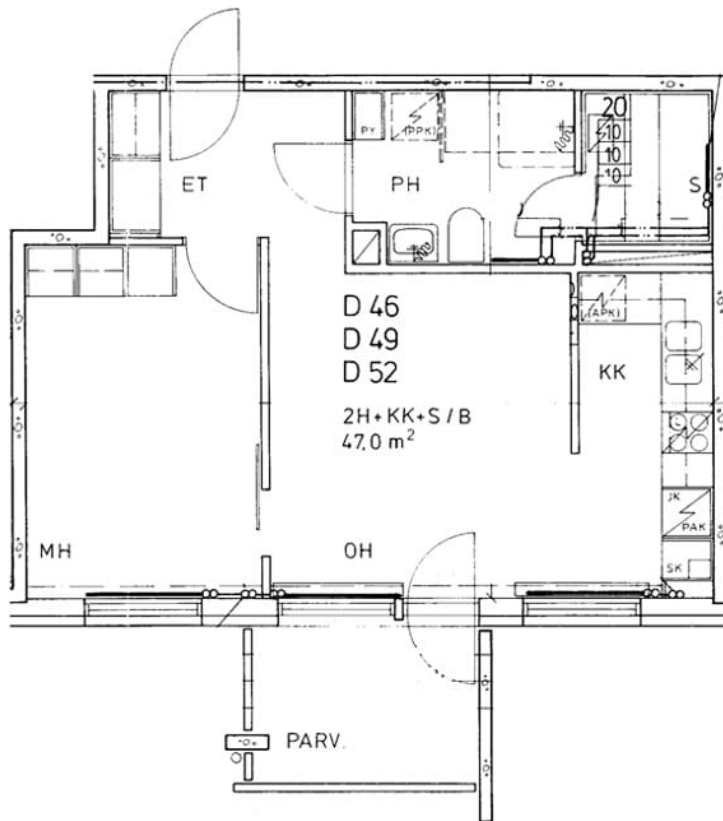
Sihtikuja 1 D 46 / pohjakuva
