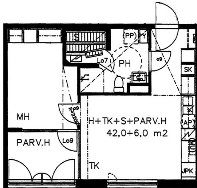
Valssikuja 1 A 5 / pohjakuva Not in scale
