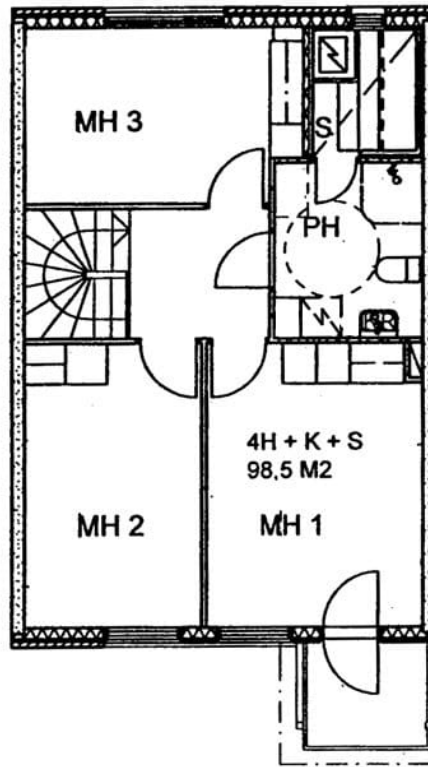
Hiilitie 7 A 2 / Pohjakuva Not in scale
