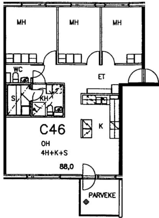
Viidakkopliku 4 C 46 / pohjakuva Not in scale
