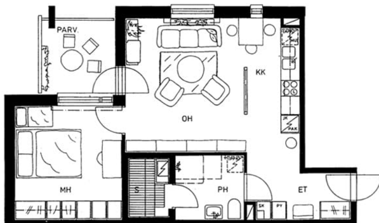
Kuorimokatu 2 B 25 / pohjakuva
