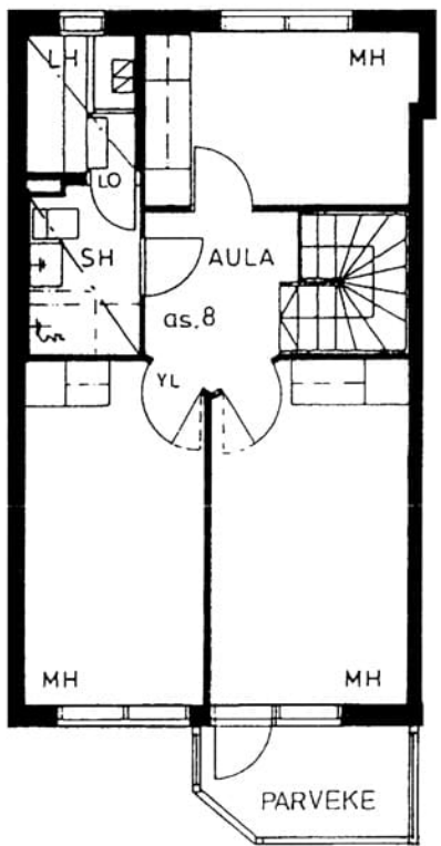
Solmukuja 4 C 8 / pohjakuva 2. kerros
