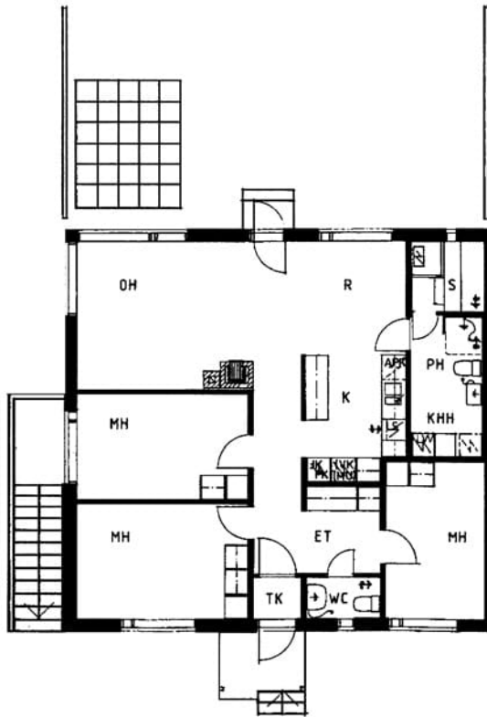
Kuismakuja 4 B 2 / pohjakuva Ei mittakaavassa
