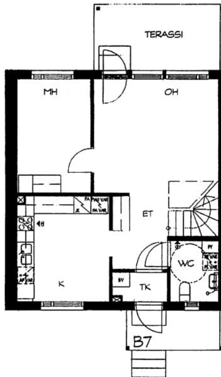
Voudinkuja 3 B 7 / pohjakuva 1.kerros Not in scale
