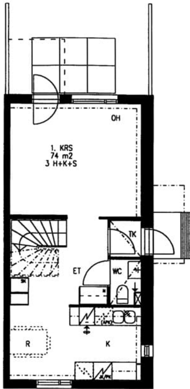
Andersinkatu 5 E 17 / pohjakuva 1.kerros Ei mittakaavassa
