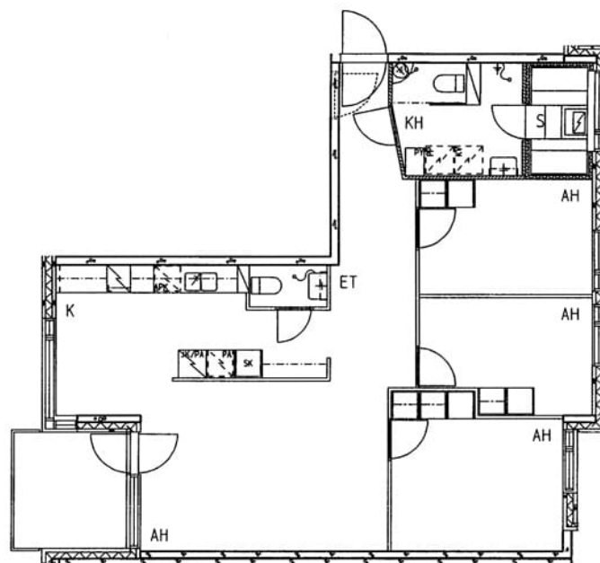
Takomotie 25 C 56 / pohjakuva
