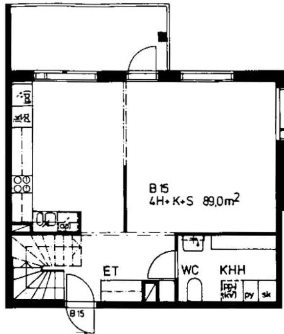
/ pohjakuva 1.kerros Ei mittakaavassa
