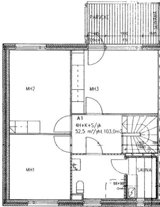
Rauduntie 12 B 3 / pohjakuva 2. kerros Not in scale
