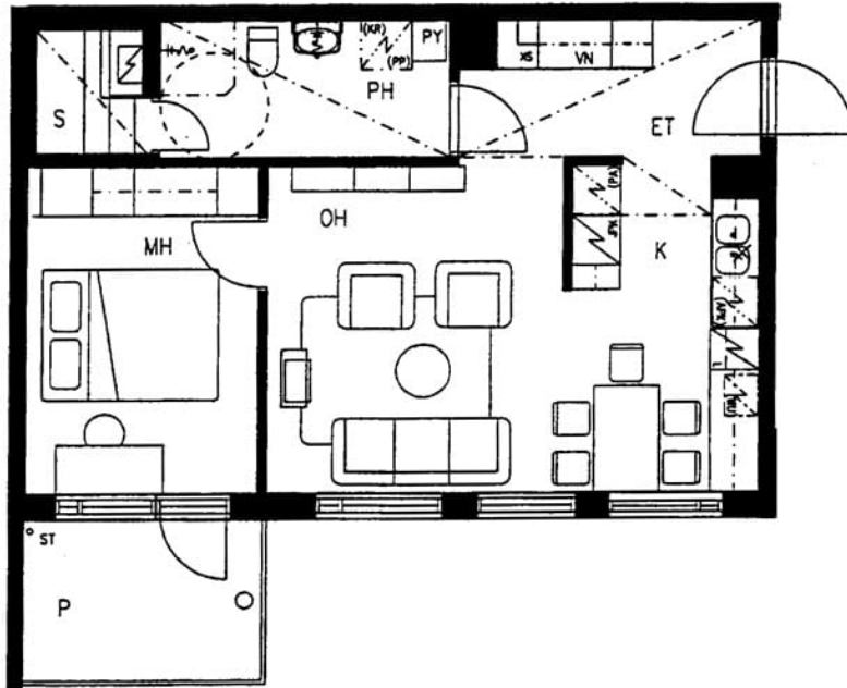
Suuruspääntie 9 A 16 / pohjakuva
