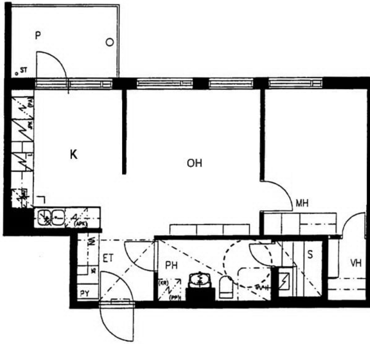
Suuruspääntie 9 A 3 / Pohjakuva Not in scale
