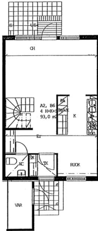
Lehtimäenkuja 4 B 6 / pohjakuva 1. kerros
