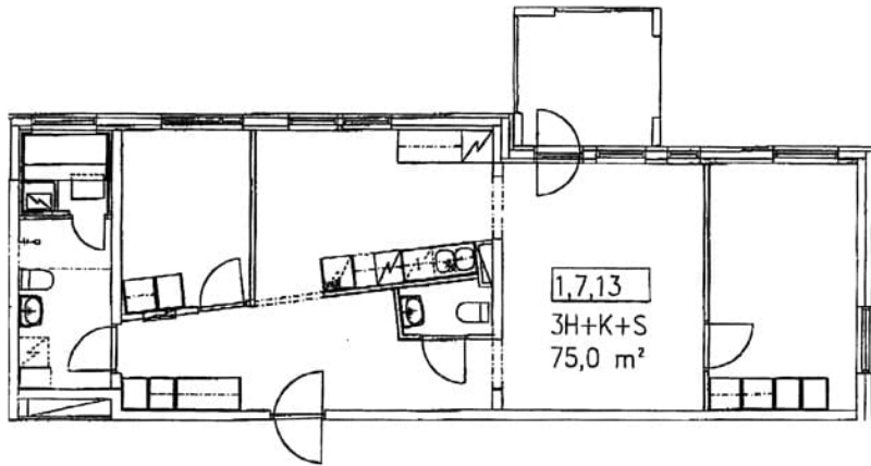
Kangastuvankatu 8 A 13 / pohjakuva Ei mittakaavassa
