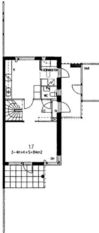
Rapolantie 8-10 F 17 / pohjakuva 1. kerros
