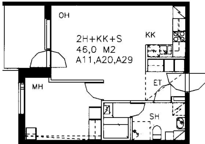
Karsikkokuja 6 A 20 / pohjakuva
