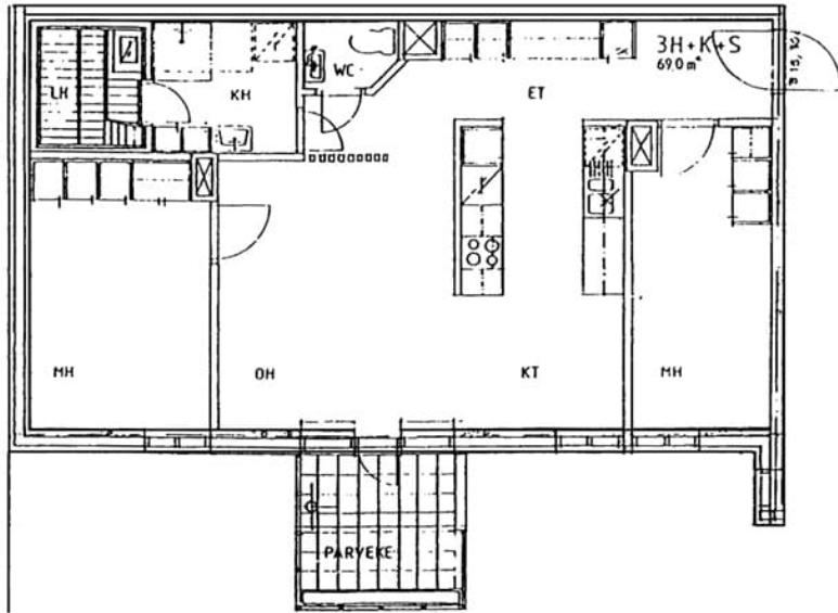
Saimaankatu 58 B A 26 / pohjakuva
