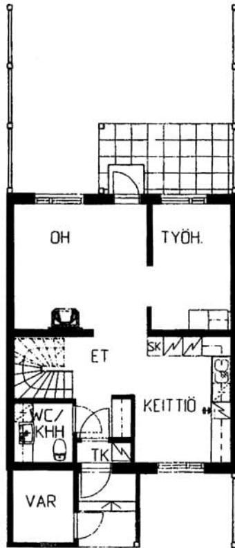
Kauniskuja 1 G 3 / pohjakuva 1. kerros
