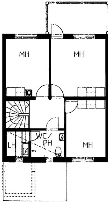
Kauniskuja 1 G 3 / pohjakuva 2. kerros Not in scale
