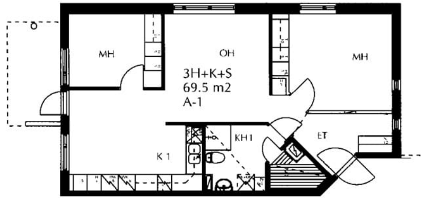
Krakantie 2B A 1 / pohjakuva
