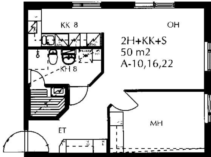
Krakantie 2B A 10 / pohjakuva Ei mittakaavassa
